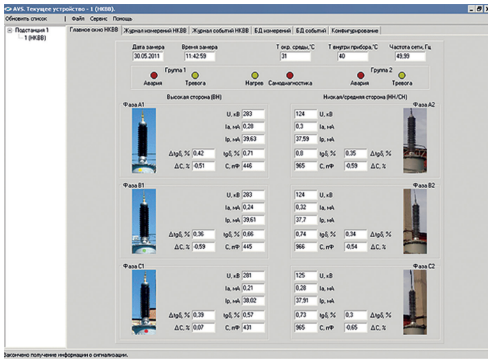
Интерфейс сервисной программы для работы с НКВВ
