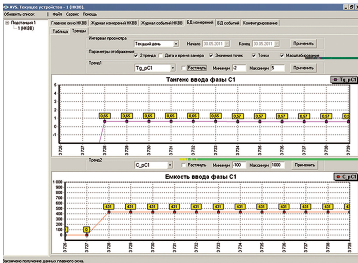
Тренды контролируемых параметров
